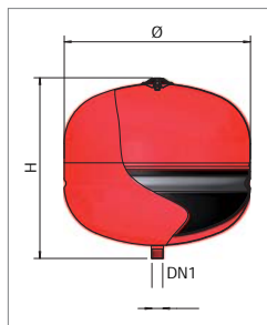
ERCE 35 - 50
