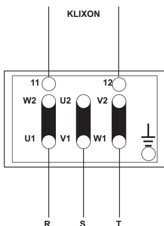
Collegamento a triangolo alla morsettiera di motori 400/400 V YA. velocità alta.
