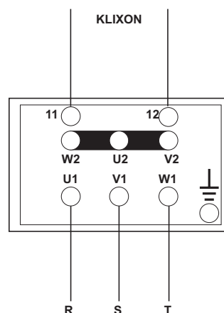
Collegamento a stella alla morsetti di motori 400/400 V YΔ. velocità bassa.
