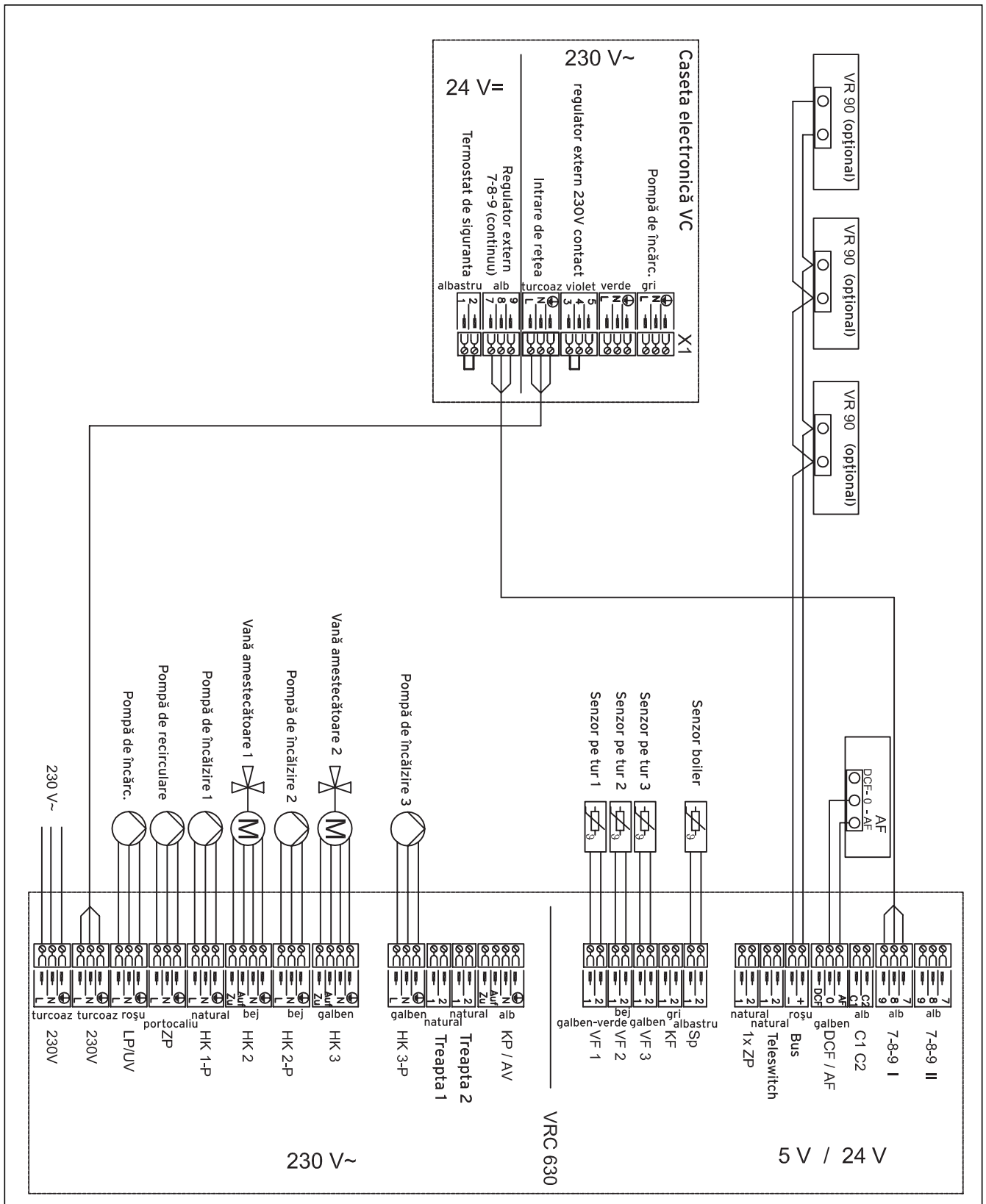
Fig. 4.11 Cablajul de conectare VRC 630 la aparatul vertical
