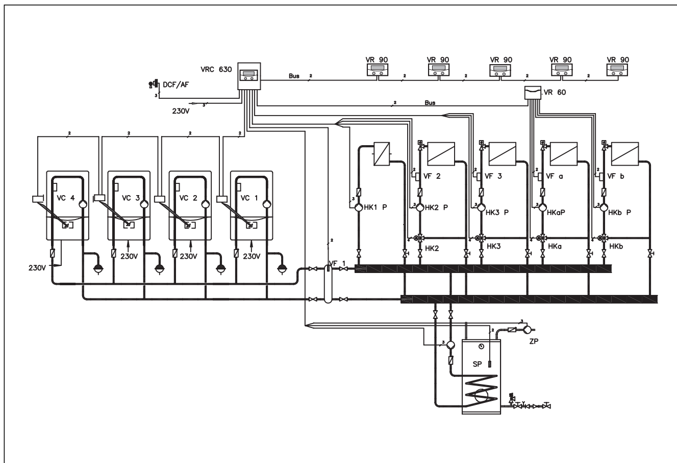
Fig. calorMATIC 630 cu 5 circuite de încălzire și 4 VC 466
