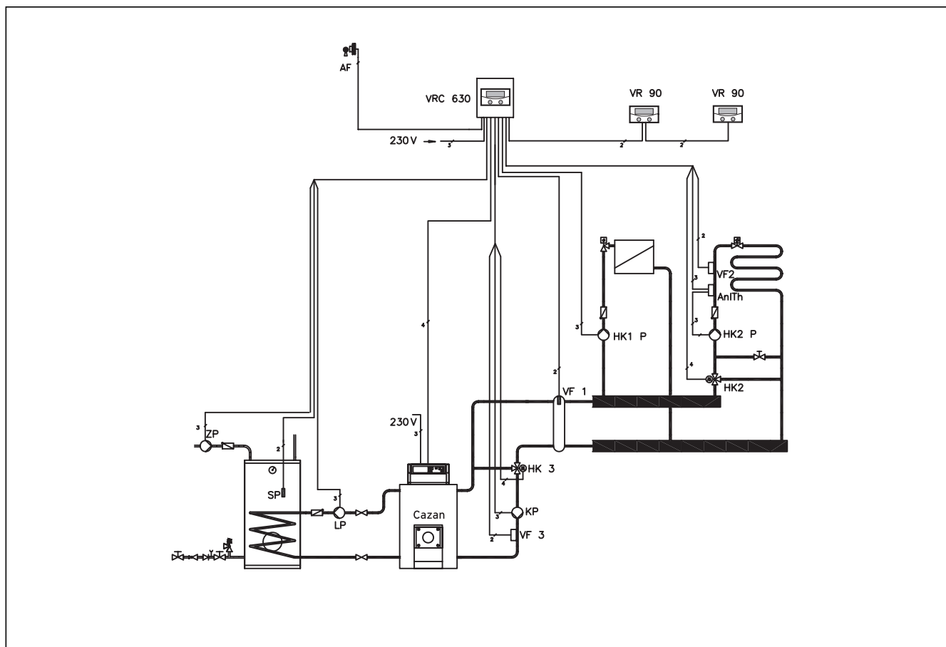
Fig. 4.12 VRC 630, cu ridicare a temperaturii pe retur
