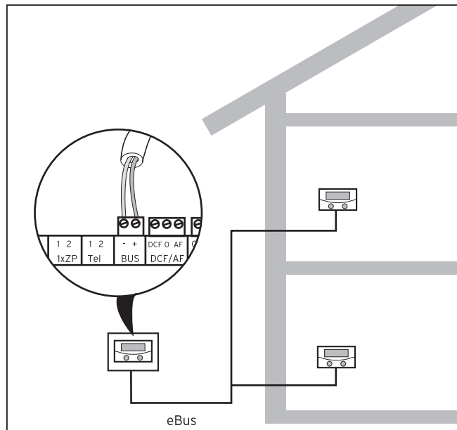
Fig. 4.17 Conectarea aparatului de comandă de la distanță
