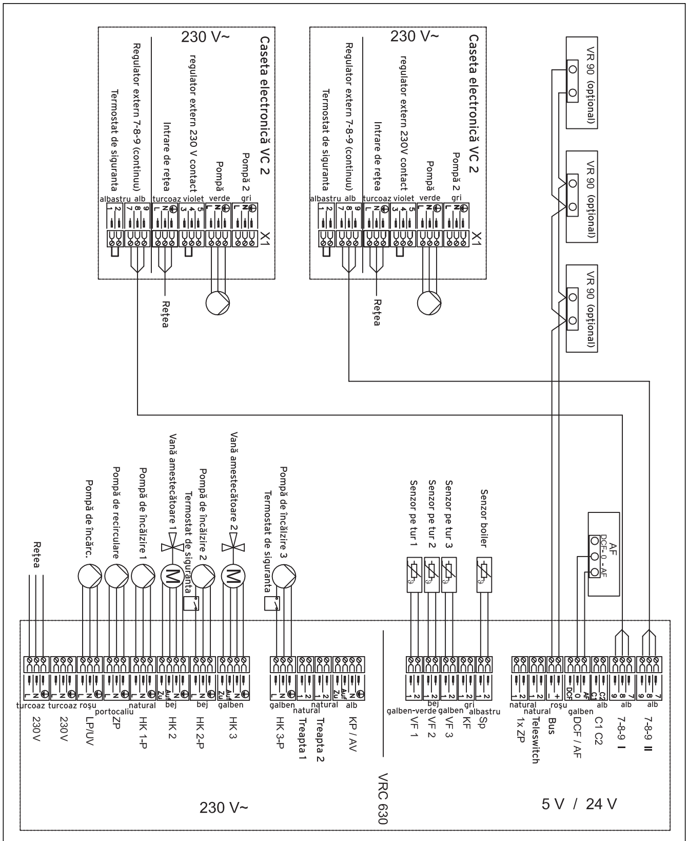
Fig. 4.7 Cablajul de conectare VRC 630, 2...VC, 3 HK, VIH
