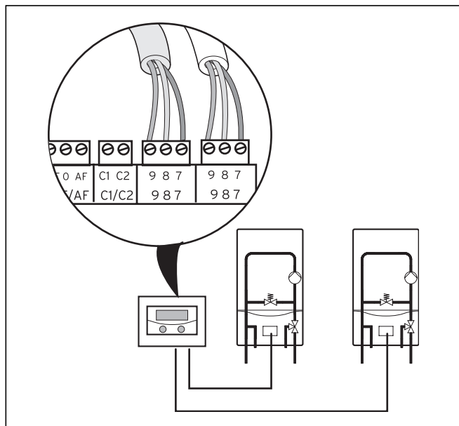
Fig. 4.19 Racordarea celei de-a doua succesiune de trepte (cascadă).
