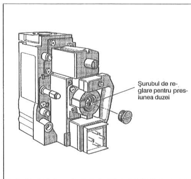
Fig. 46: Armătura arzătorului de gaze Honeywell VR 4601
