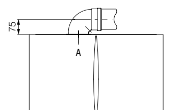
Quota kit concentrico Ø 60/100
