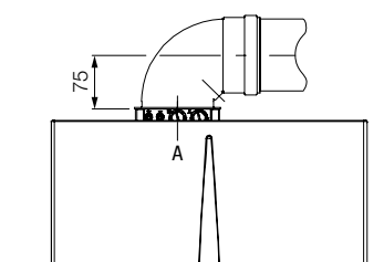
Quota kit concentrico Ø 60/100
