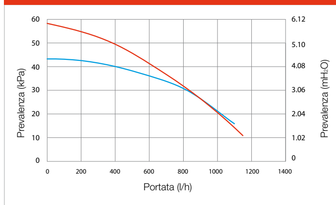
Grafico portata e prevalenza VICTRIX Mini 24 kW
