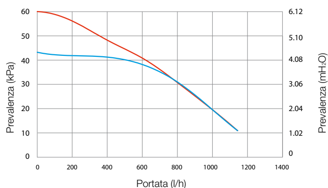
Grafico portata e prevalenza VICTRIX Intra 26 kW/Plus
