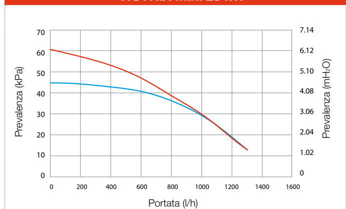
Grafico portata e prevalenza VICTRIX Mini 28 kW
